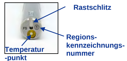
FS Sender mit geringer Reichweite mit Nahaufnahme der vorderen Endkappe
