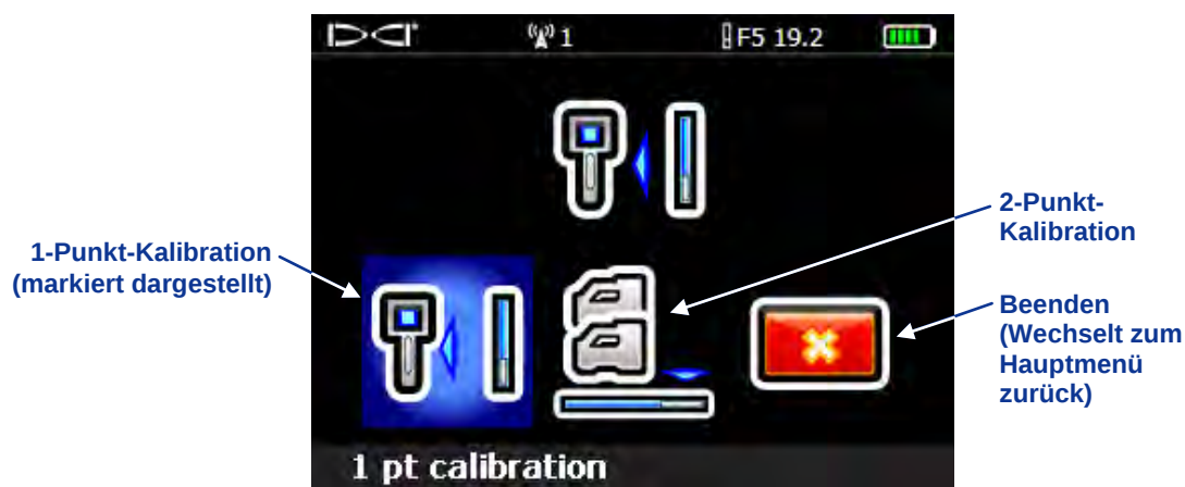
Kalibrationsmenübildschirm des Empfängers
