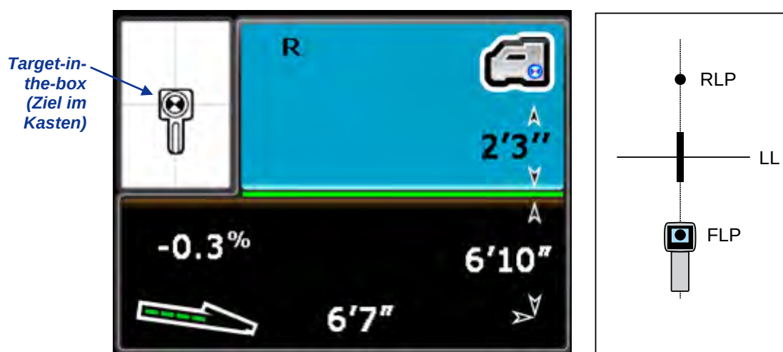
Tiefenmodus-Bildschirm des Empfängers (am FLP mit aktivierter HÜG)
