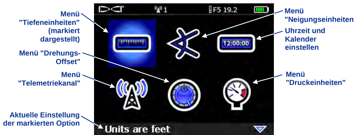
Menü "Einstellungen" des Empfängers, erster Bildschirm
