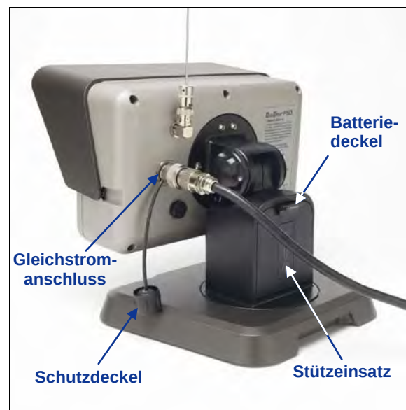
Gleichstromkabel und Stützeinsatz in FSD Fernanzeige eingebaut
