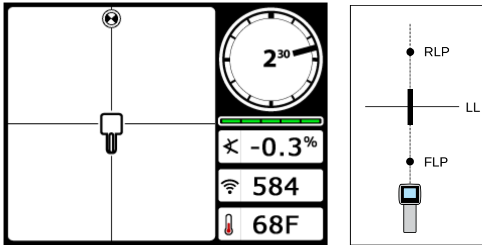
Bildschirm für "fliegendes" Verfolgen des Empfängers
