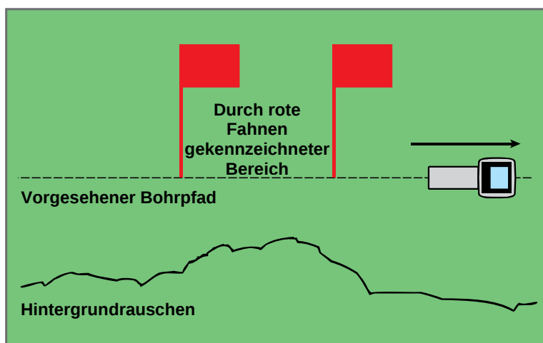
Einpersonenprüfung der Hintergrundsignalstärke (kein Sender)
