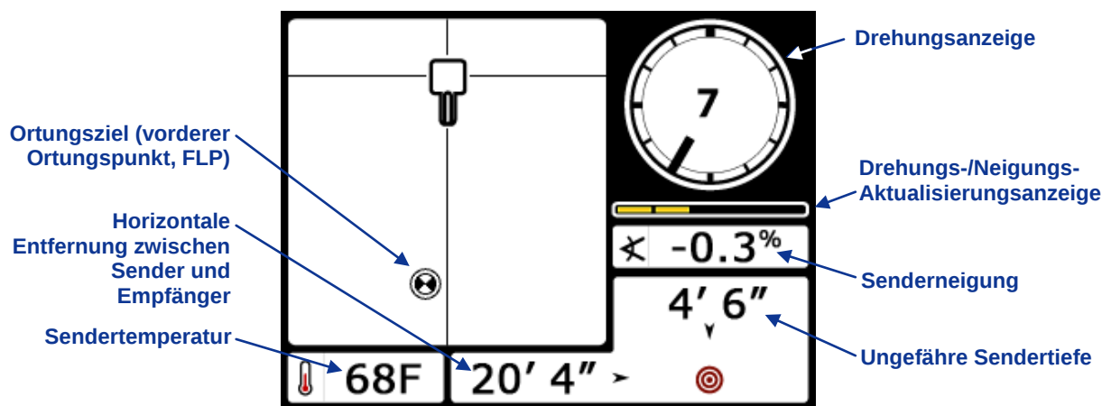
Zielansteuerungs-Bildschirm im Ortungsmodus
