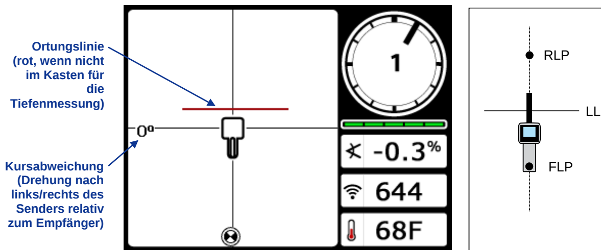
Ortungsmodus-Bildschirm des Empfängers (bei Annäherung an die LL)
