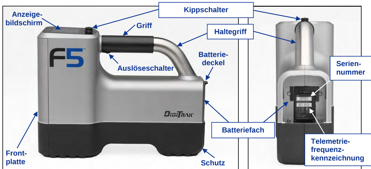
F5 Empfänger – Ansicht von der Seite und von hinten
