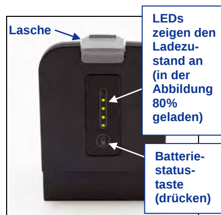
F Series Batterie
