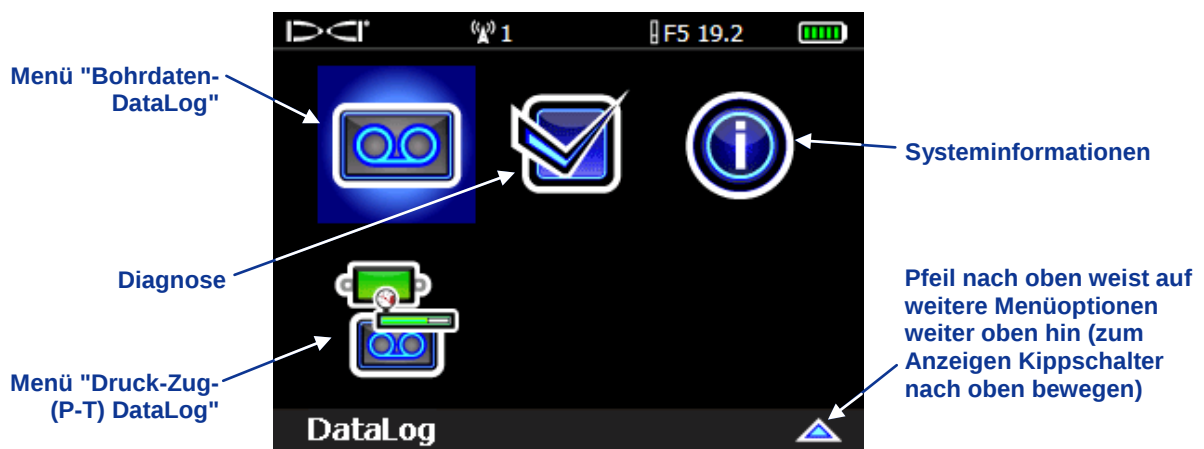
Hauptmenü des Empfängers, zweiter Bildschirm
