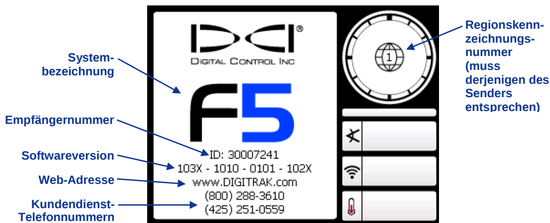
Empfänger-Startbildschirm
