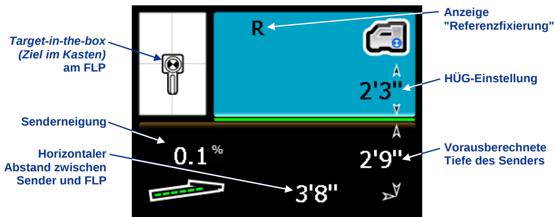
Bildschirm für die vorausberechnete Tiefe des Empfängers am FLP bei aktivierter HÜG (Auslöser gedrückt)
