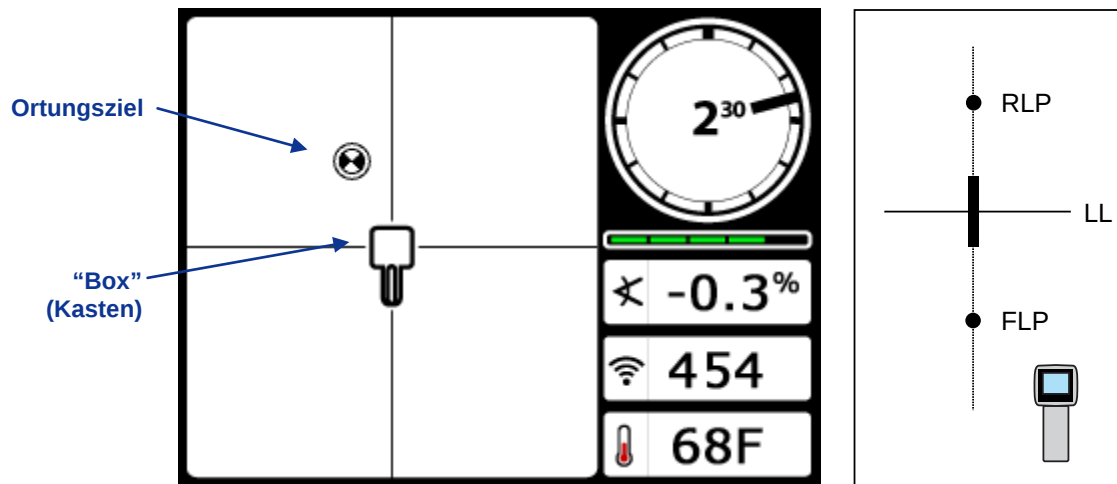
Ortungsmodus-Bildschirm des Empfängers
