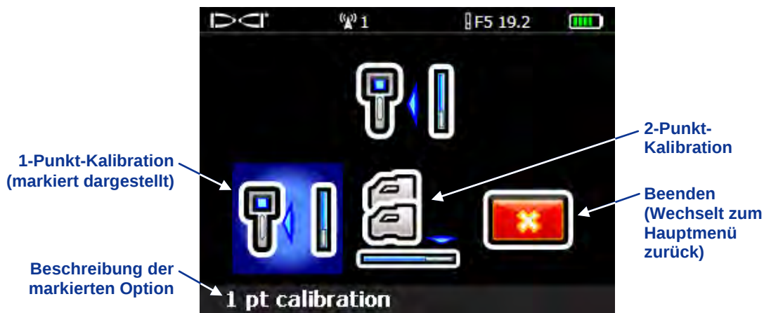
Menü "Kalibration" des Empfängers
