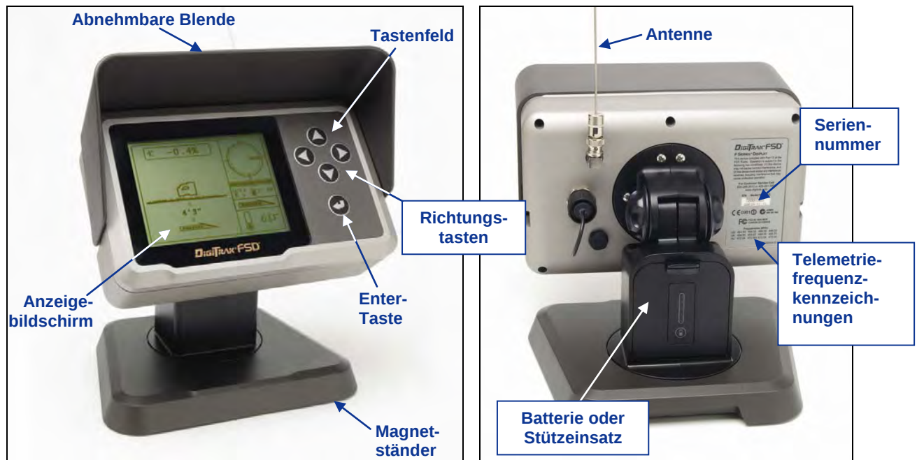
DigiTrak F Series Anzeig (FSD) Vorne und Hinten
