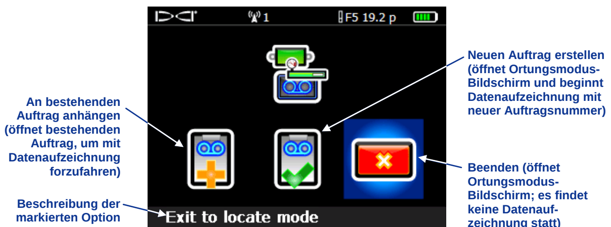
Menü "Druck-Zug-DataLog Aufzeichnung starten"
