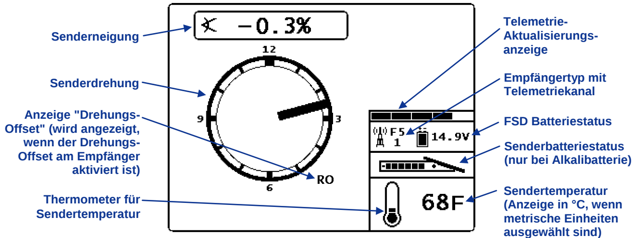
FSD Hauptanzeigebildschirm
