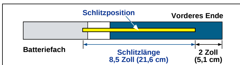
Gehäuseschlitzanforderungen für Sender mit großer Reichweite
