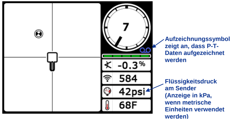
Ortungsmodus-Bildschirm mit Flüssigkeitsdruckdaten (Auslöser aus)
