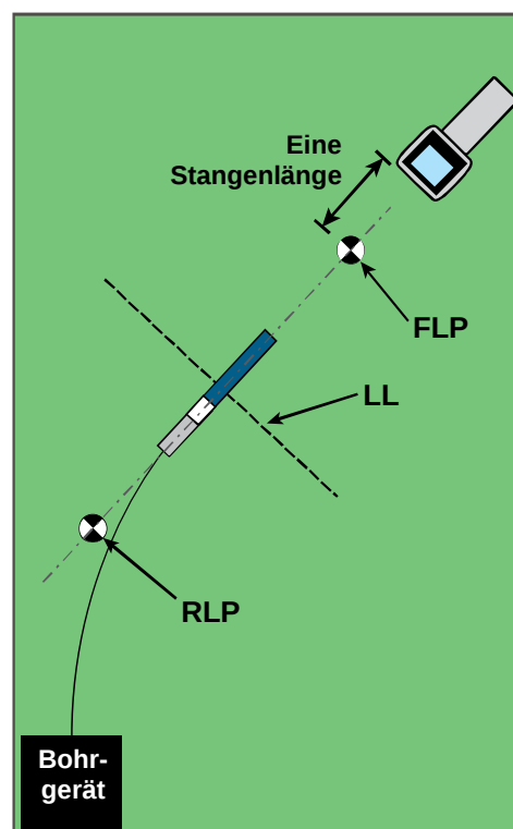
"Fliegendes" Verfolgen bei gekrümmtem Pfad
