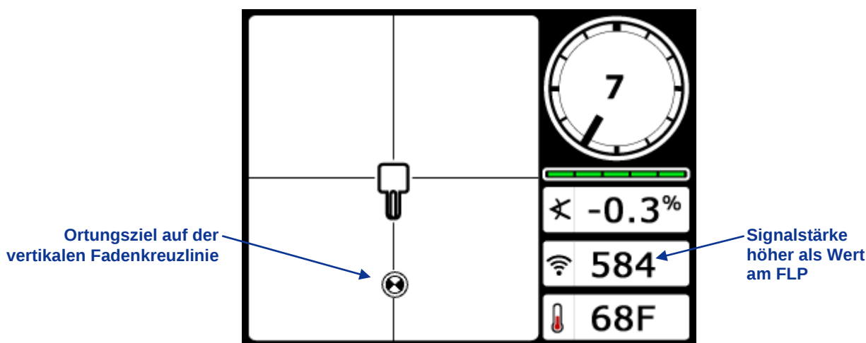
Ortungsmodus-Bildschirm des Empfängers (FLP hinter Empfänger, der sich auf die LL zu bewegt)
