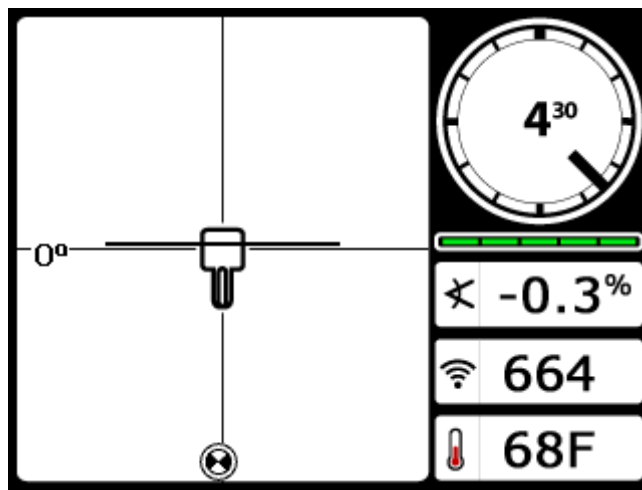
Tiefenmodus-Bildschirm des Empfängers (an der LL)
