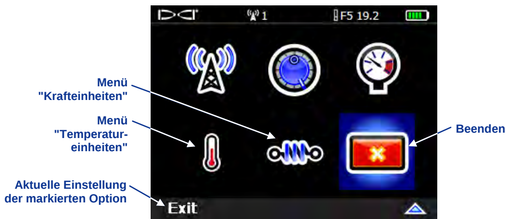
Menü "Einstellungen" des Empfängers, zweiter Bildschirm
