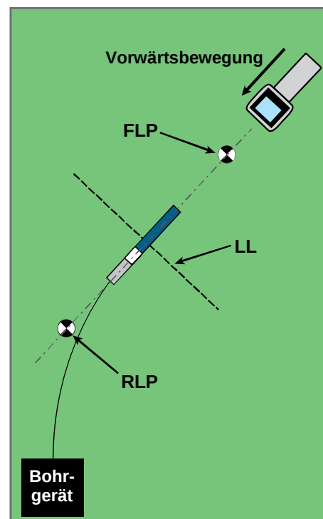
Standardortungsverfahren bei gekrümmtem Pfad
