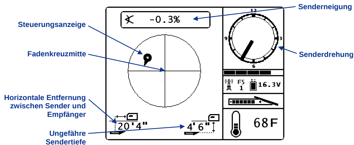
Zielansteuerung an der Fernanzeige
