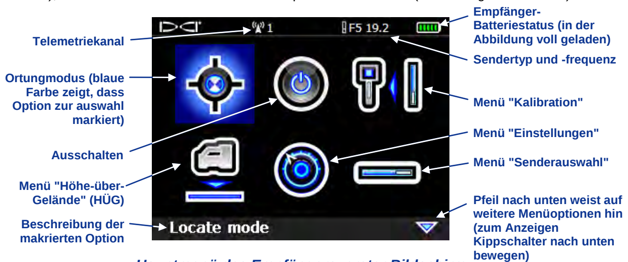
Hauptmenü des Empfängers, erster Bildschirm
