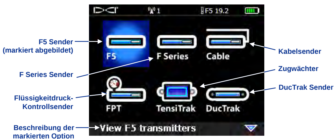
Hauptmenü "Senderauswahl"
